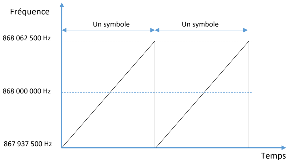
Figure 9 : Forme du symbole de base (CHIRP)
