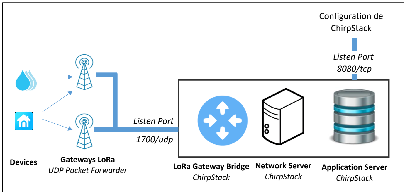
Figure 111 : Architecture globale après installation de ChirpStack
